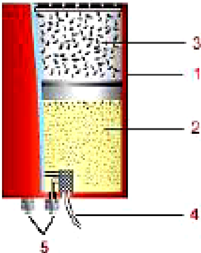
Рисунок 4.18 – Конструкция аэрозольного генератора: 1 – корпус; 2 – заряд аэрозольобразующего вещества; 3 – охладитель; 4 – огнепроводный шнур; 5 – клеммы воспламенителя
