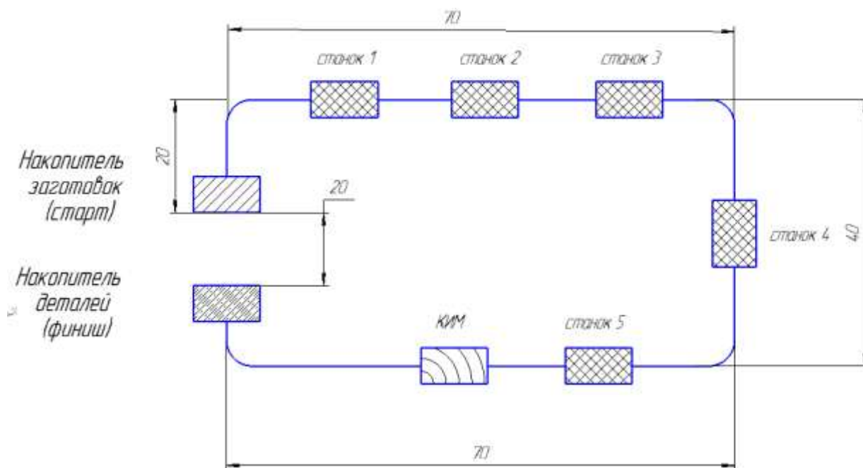
Рисунок 15. Маршрут обработки заготовки
