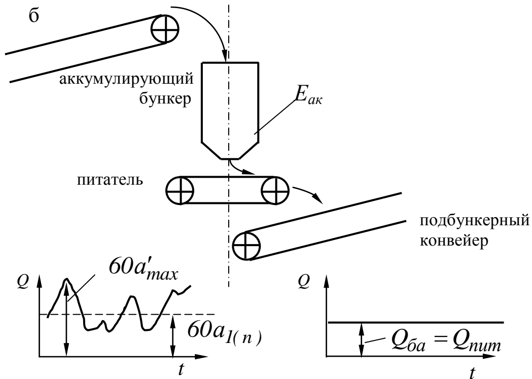
Рис. 3. Установка бункера в конвейерной линии и его влияние на сглаживание неравномерности грузопотока:
