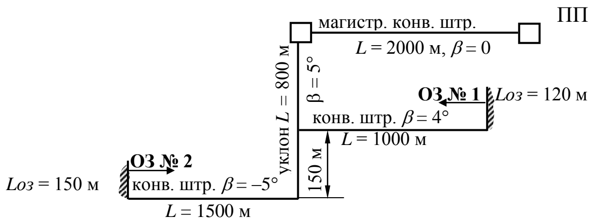
Рис. 1. Технологическая схема транспорта: а – участковая; б – участковая с магистральной выработкой; в – участковая с магистральной выработкой и аккумулирующим горным бункером
